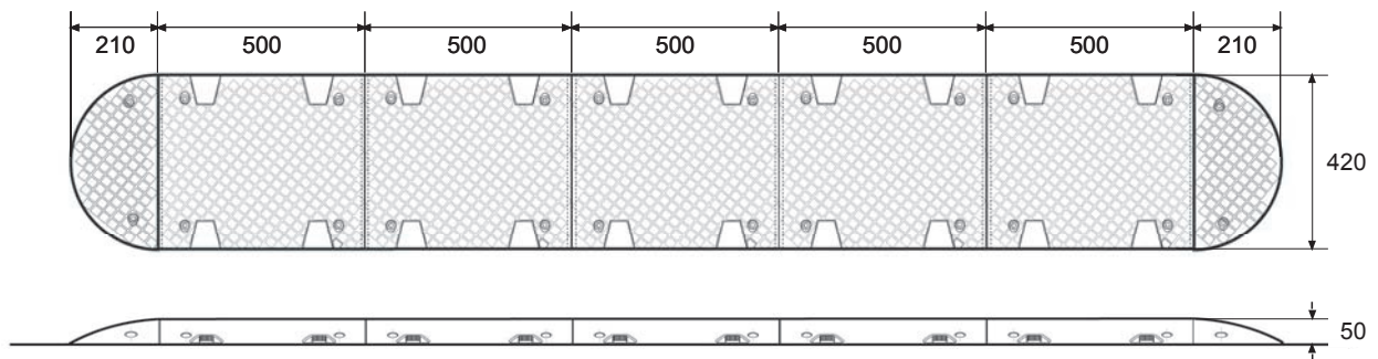
EX. PÅ SAMLET VEJBUMP
