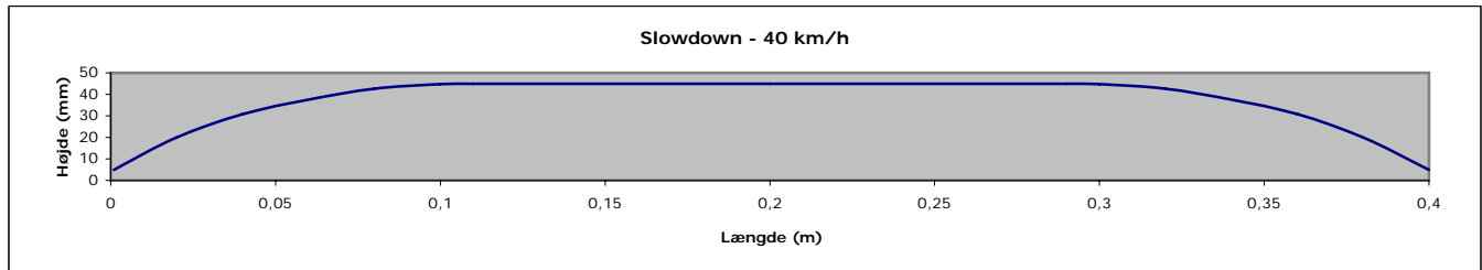
Længdeprofil bump ①
